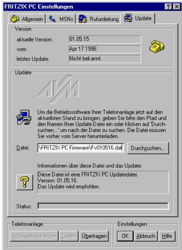
Abb. 11 Registerkarte Update
